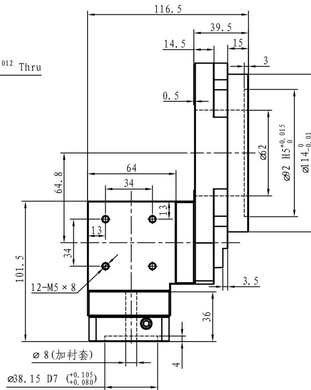
旋转部位 Rotating Part
