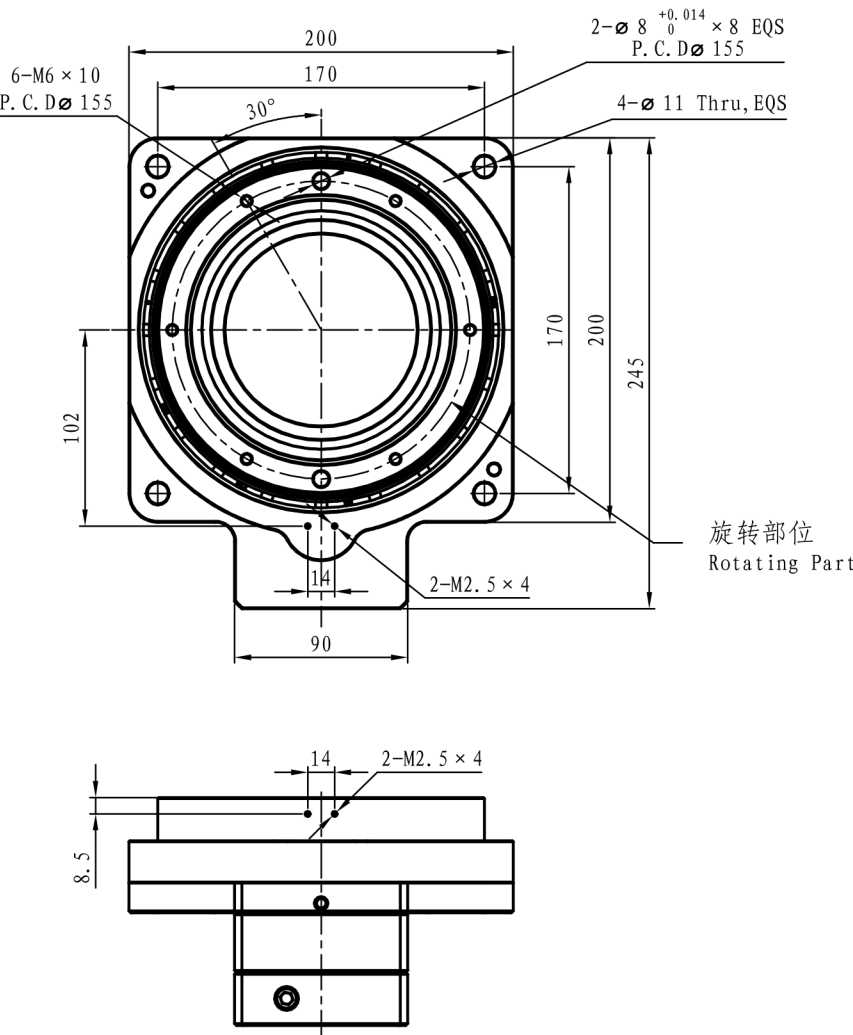
输出端 Output
