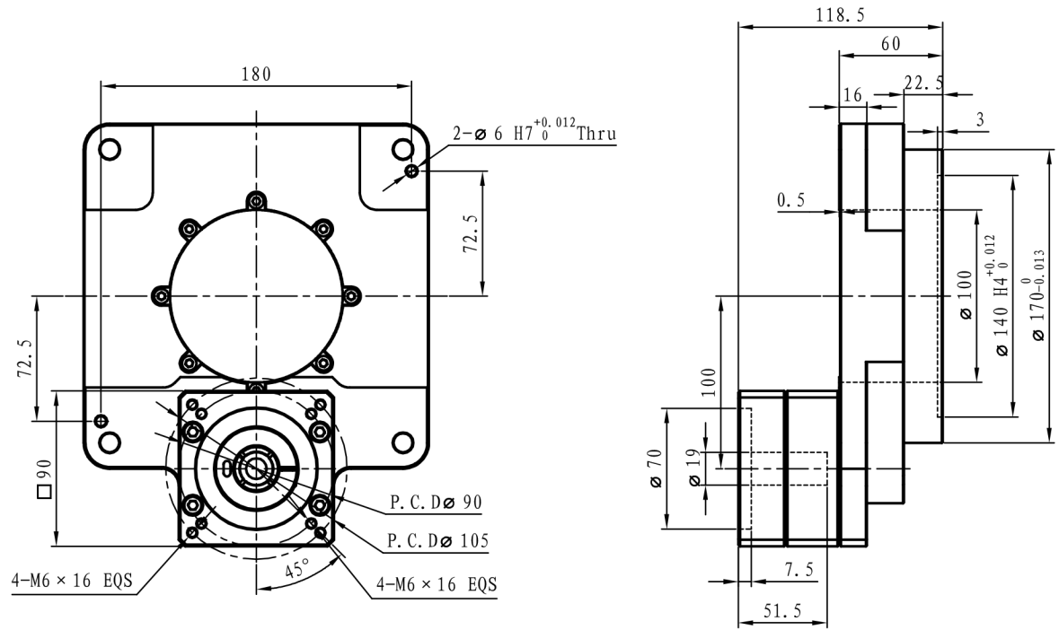
输入端 Input
