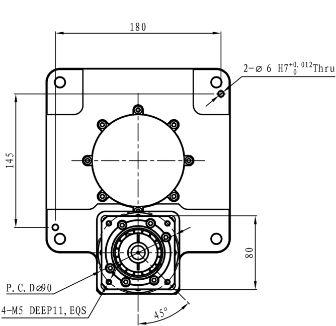
输出端 Output
