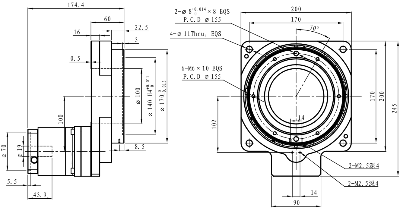
输入端 Input
